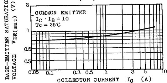
V_{BE(sat)} - I_C
