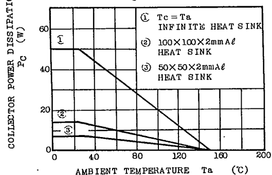
P_C - T_a
